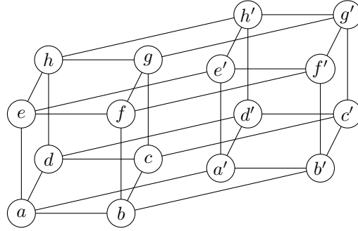
Рис. 1. Четырёхмерный куб Q_4
