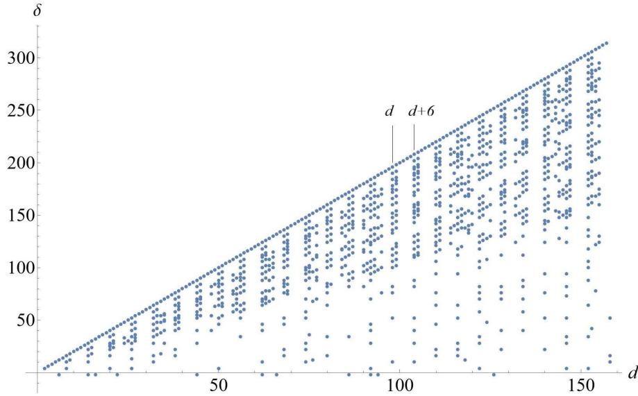
Рис. 2. Расположение порядков субоптимальных циркулянтов C(N; 1, s) в зависимости от диаметра для датасета Subopt
