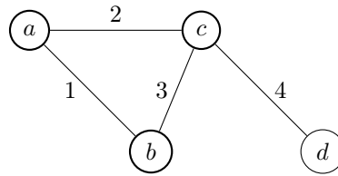
Рис. 2. Исходный граф G и покрытие C_0
